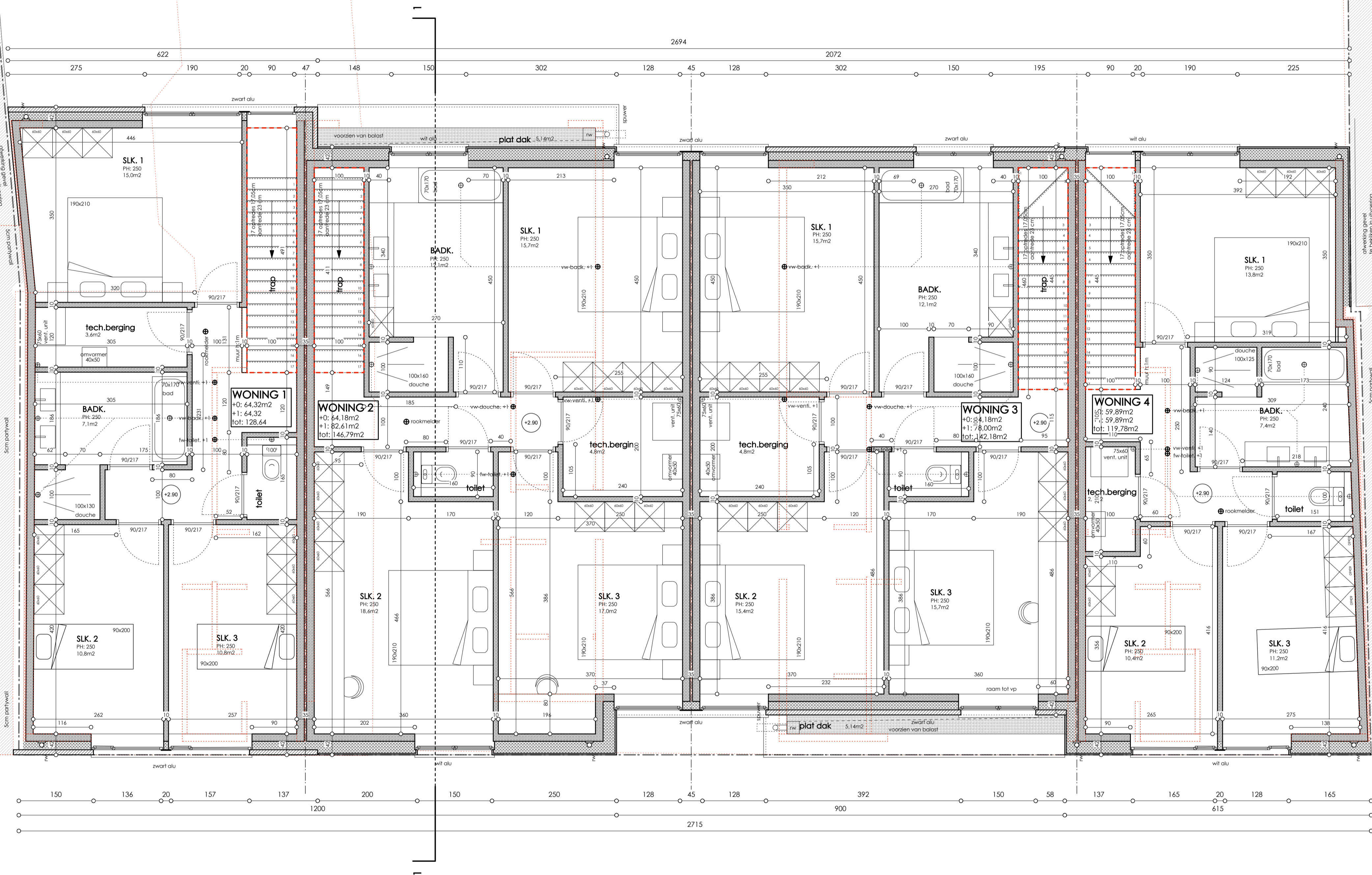
verdiepingsplan nieuwe toestand schaal 1/50
