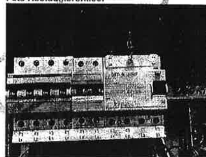
Foto Hoofddifferentieel
