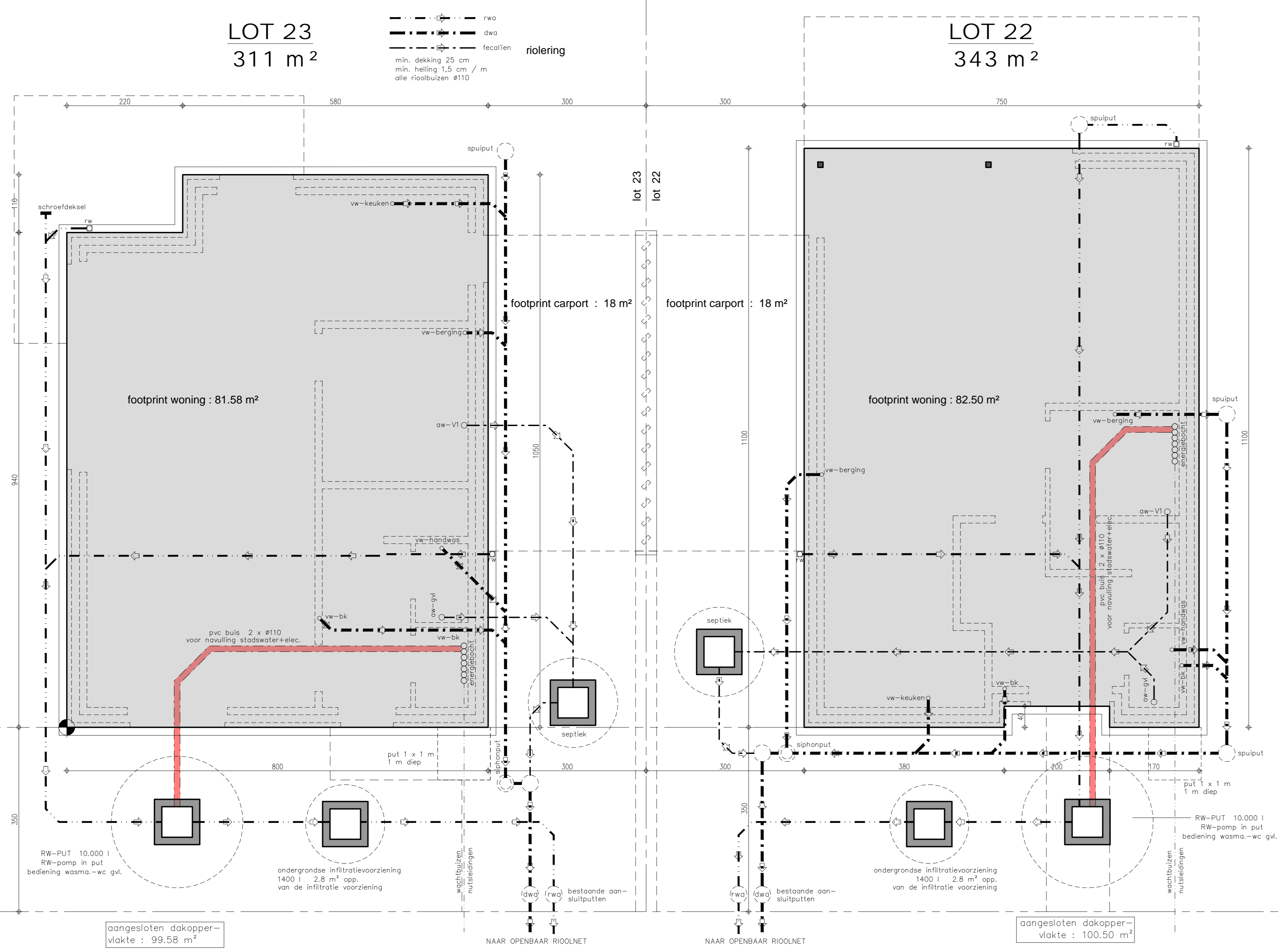
ONDERGROND - RIOLERING 1/50
