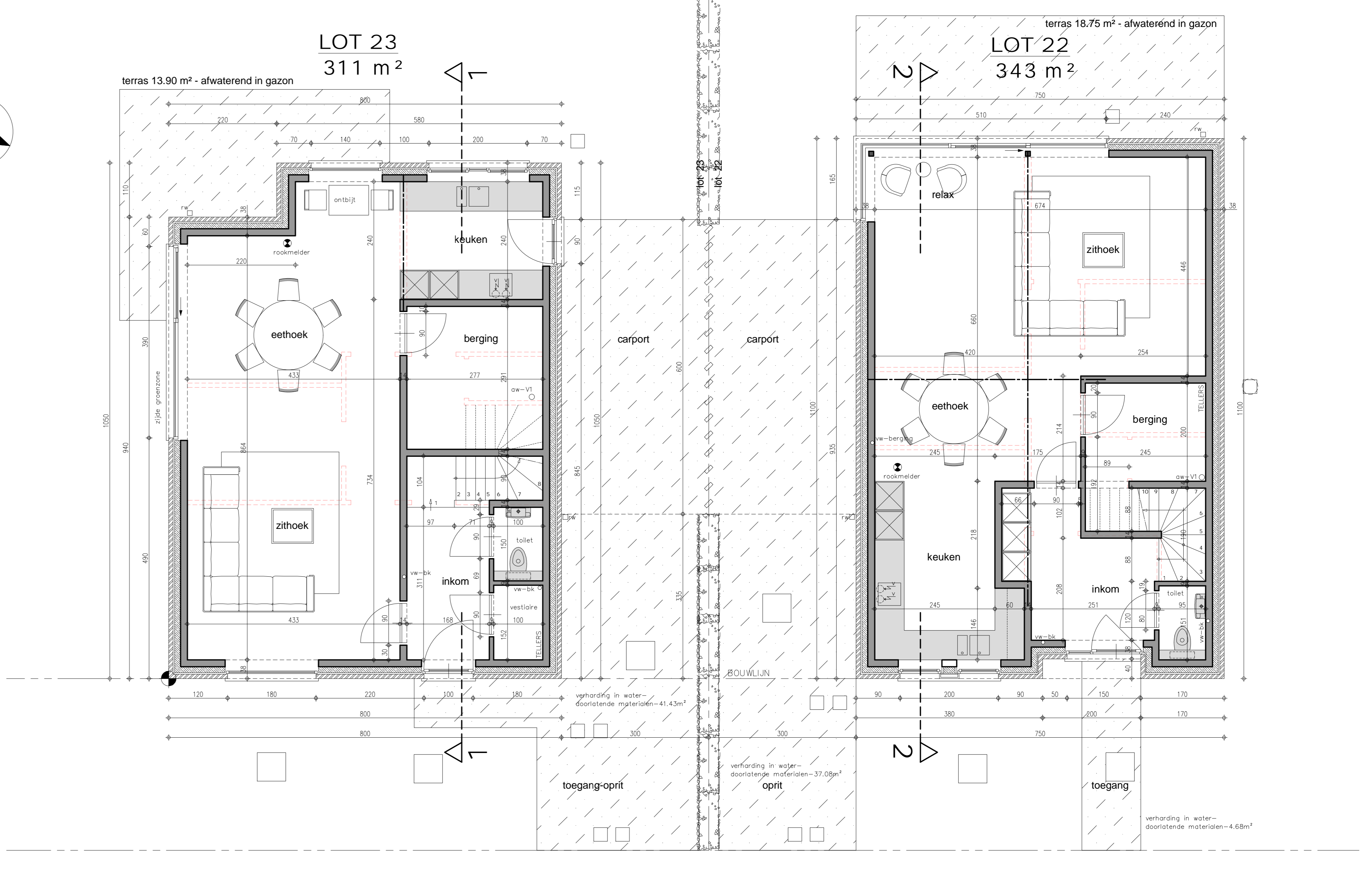
GELIJKVLOERS 1/50
