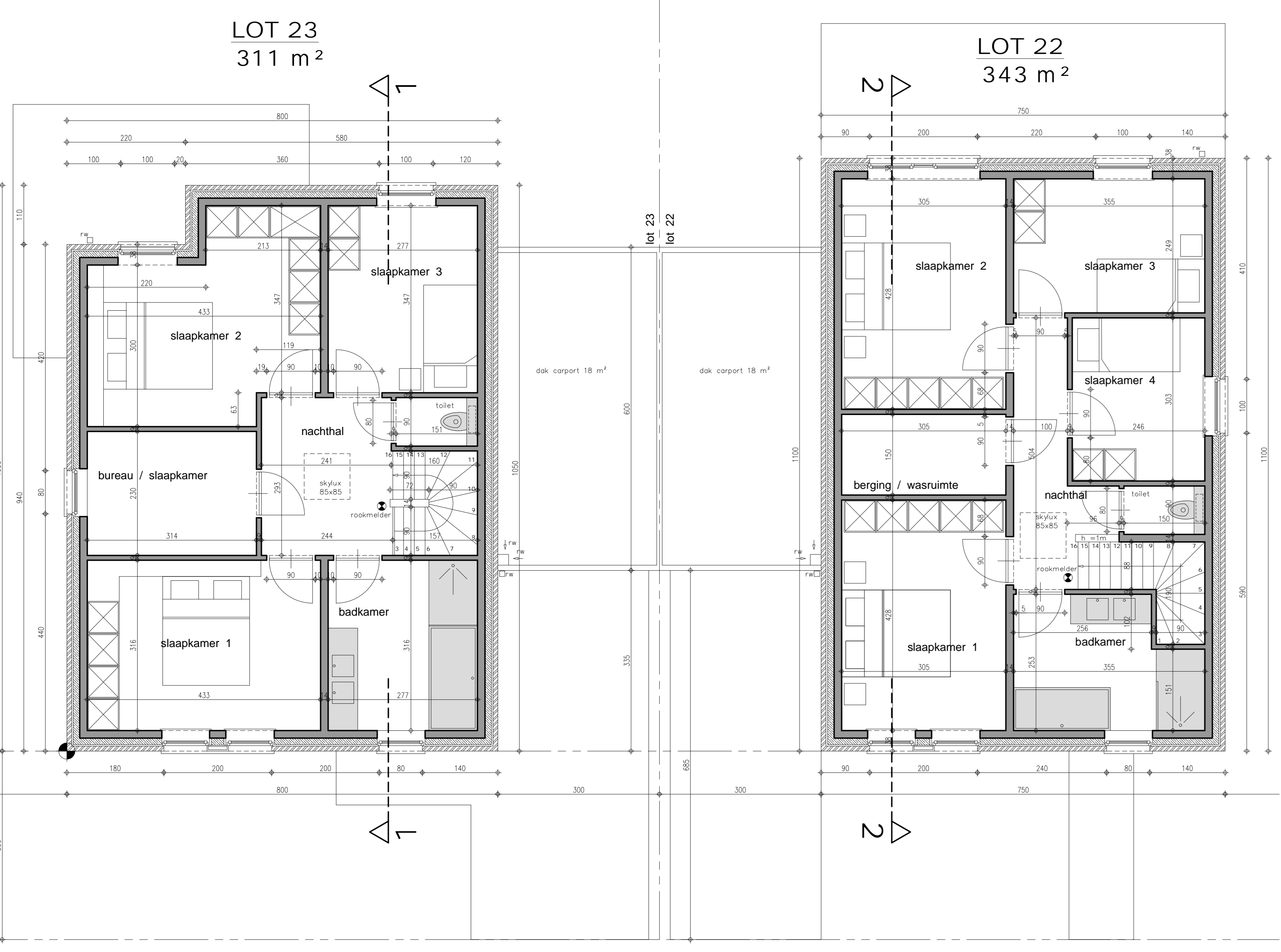
VERDIEPING 1 1/50
