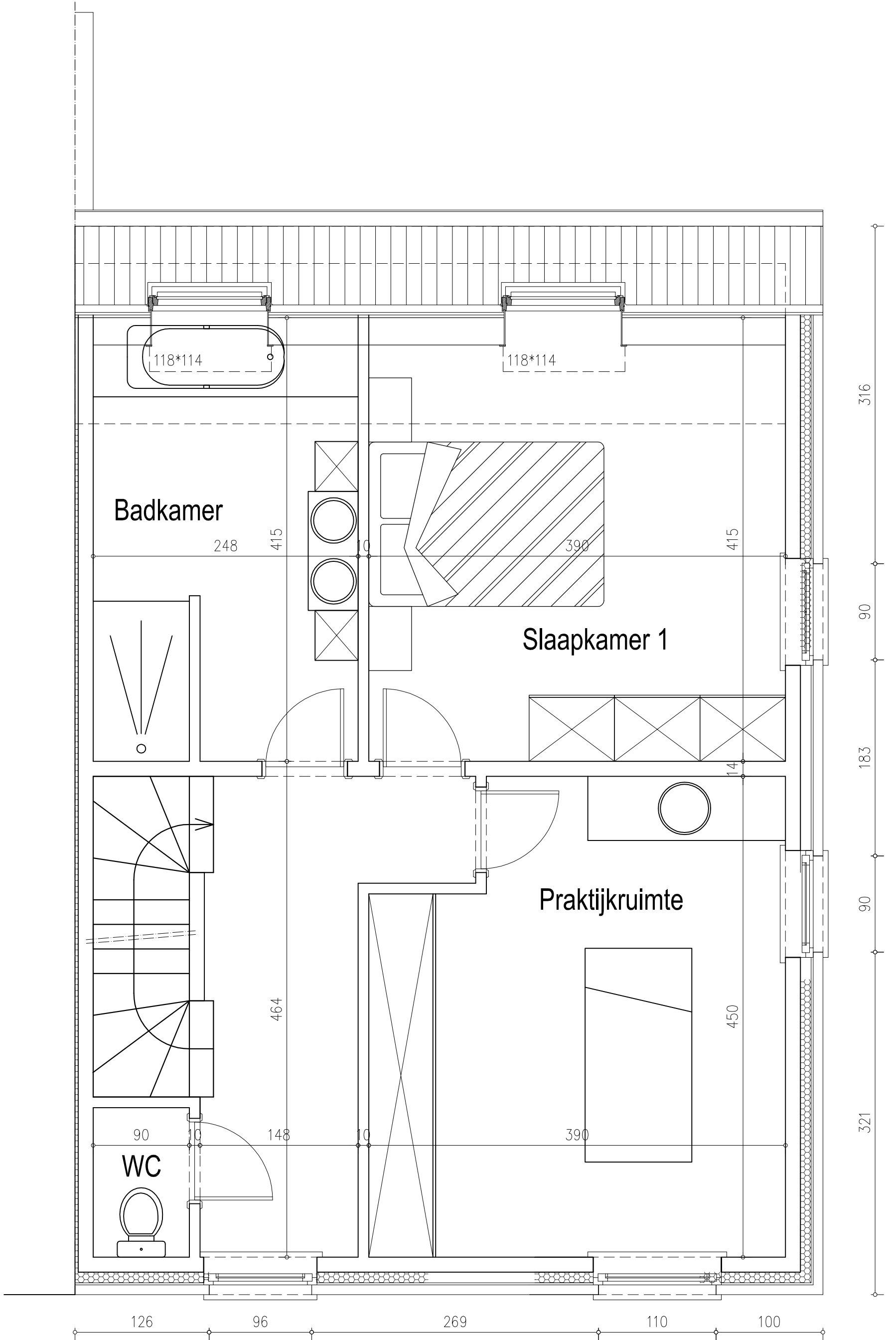
erdiepingsplan
